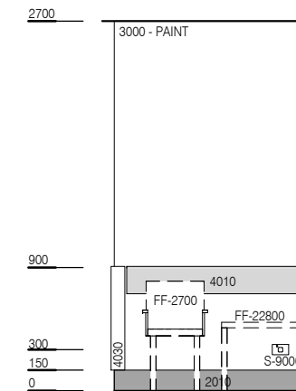
ELEVATION 3
