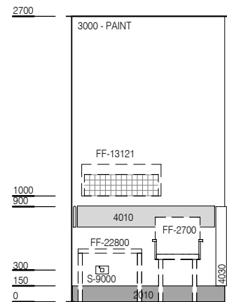
ELEVATION 2
