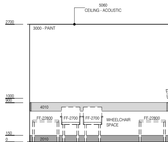
ELEVATION 1
