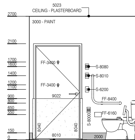
ELEVATION 3
