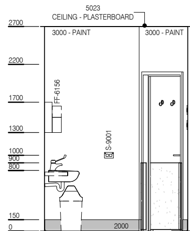
ELEVATION 1
