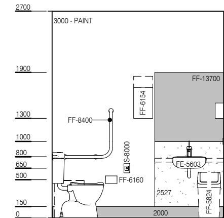
ELEVATION 4
