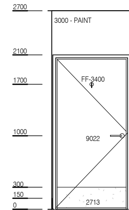
ELEVATION 3
