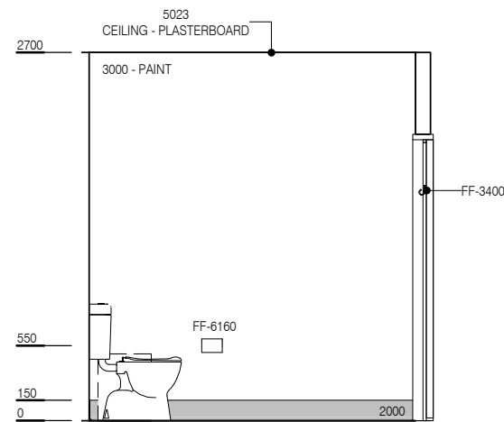
ELEVATION 2
