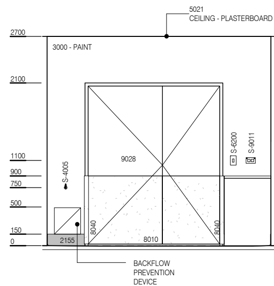
ELEVATION 1
