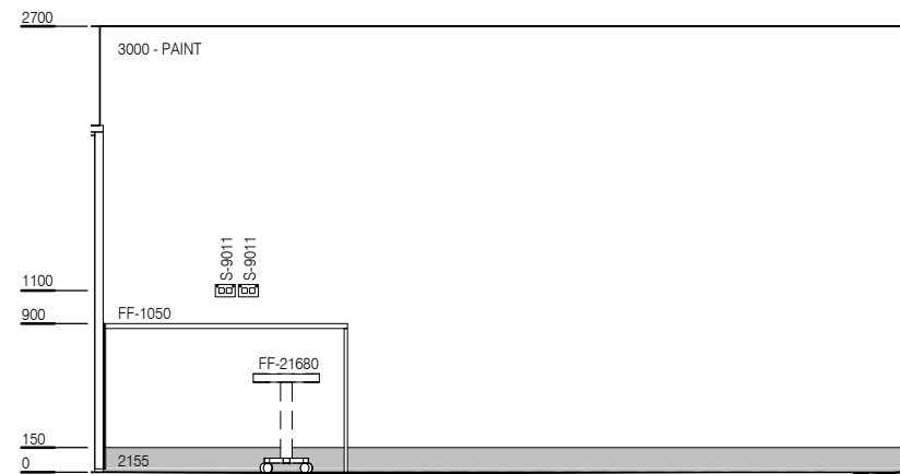
ELEVATION 2
