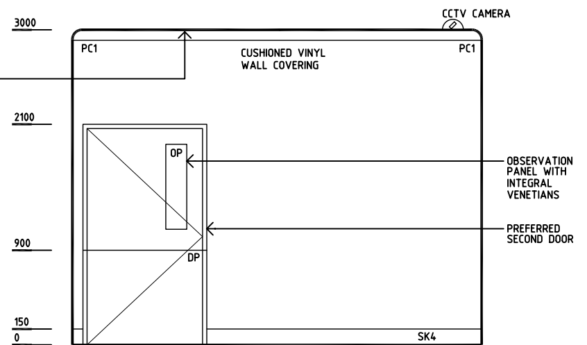
ELEVATION 2
