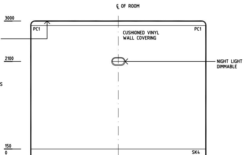
ELEVATION 2
