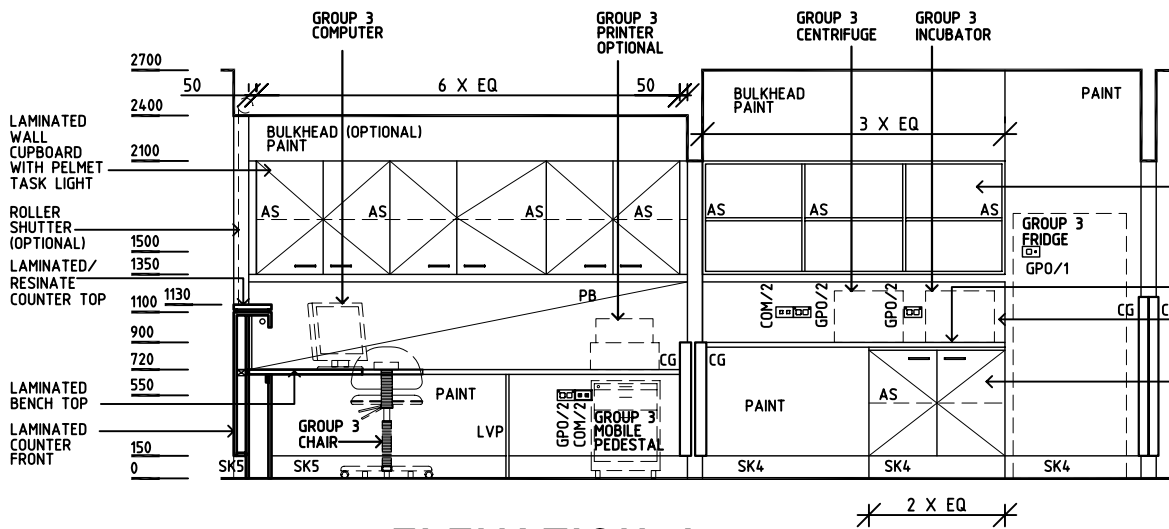
ELEVATION 1
