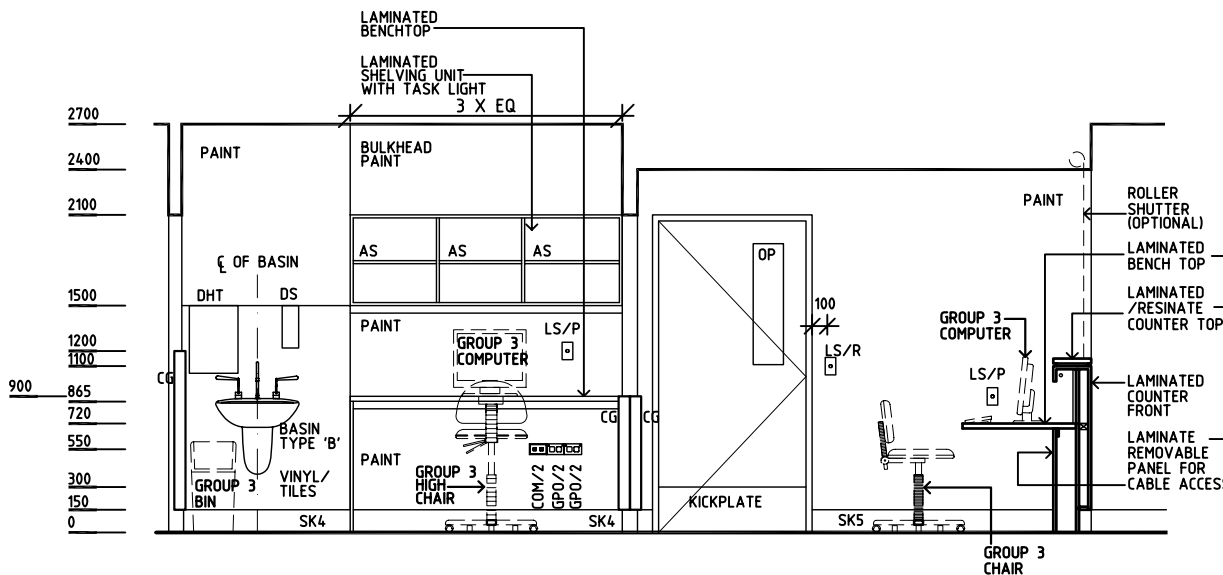
ELEVATION 3
