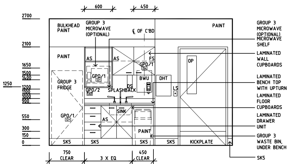
ELEVATION 3
