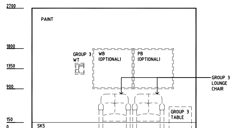
ELEVATION 4
