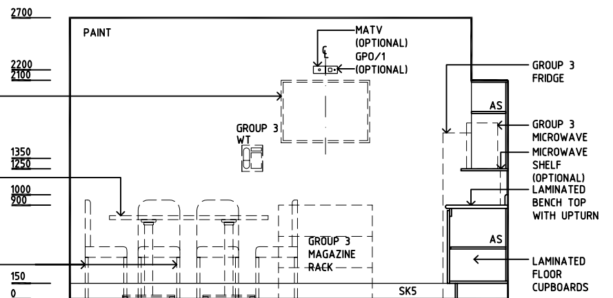
ELEVATION 2
