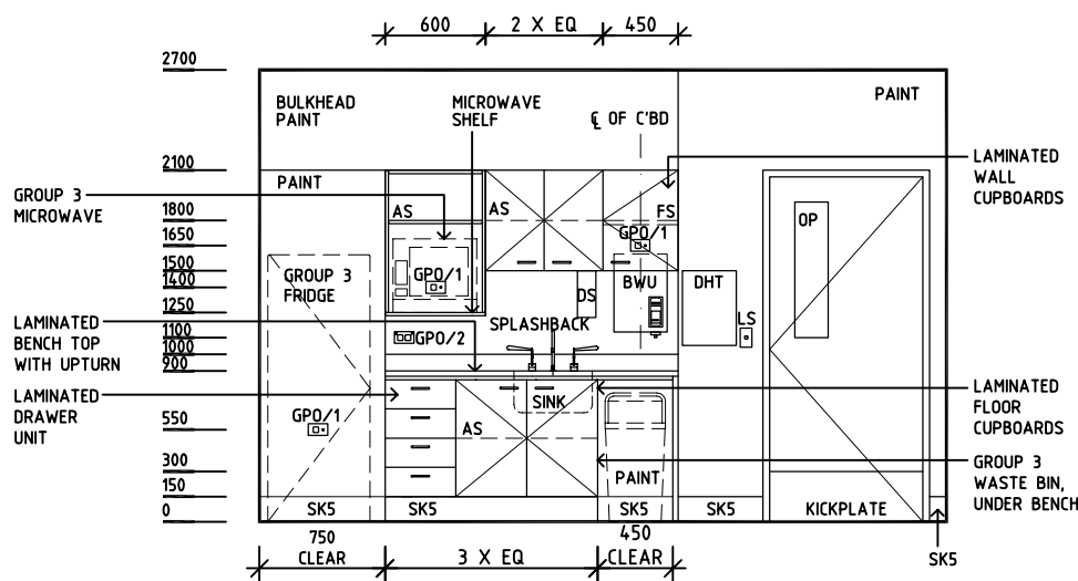
ELEVATION 3
