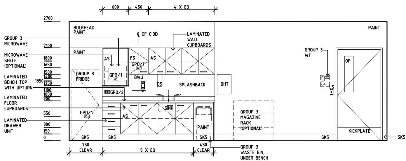
ELEVATION 3
