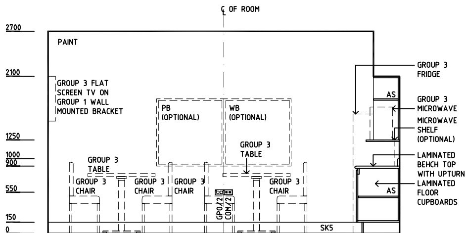
ELEVATION 2
