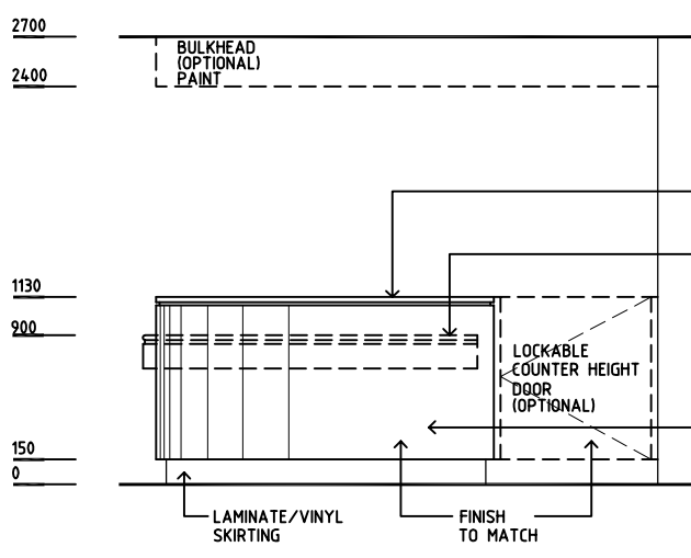
ELEVATION 1
