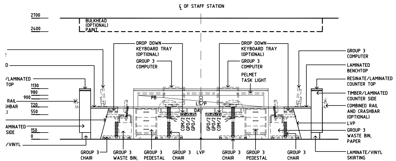
ELEVATION 5
