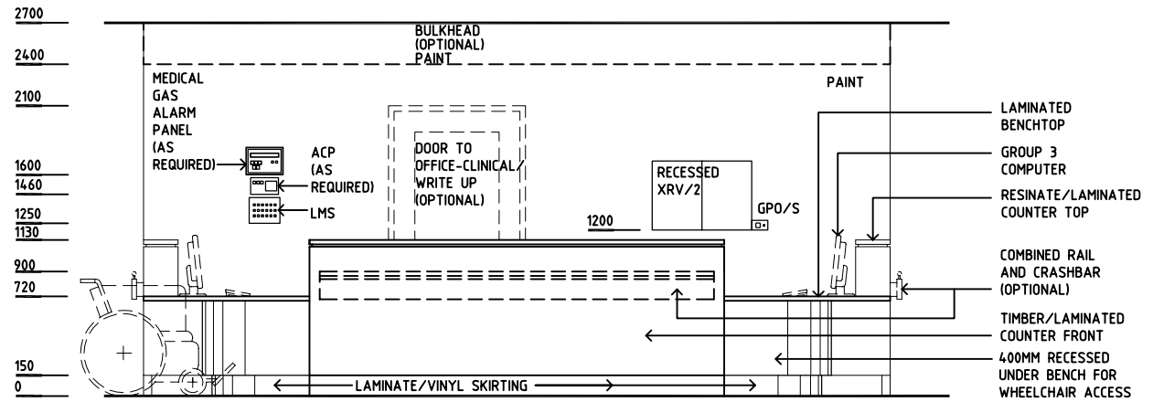
ELEVATION 2
