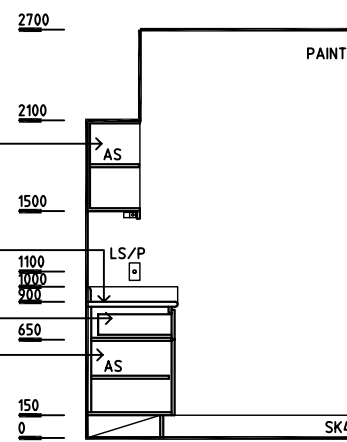
ELEVATION 2
