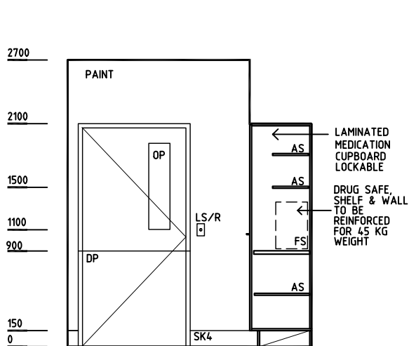
ELEVATION 3
