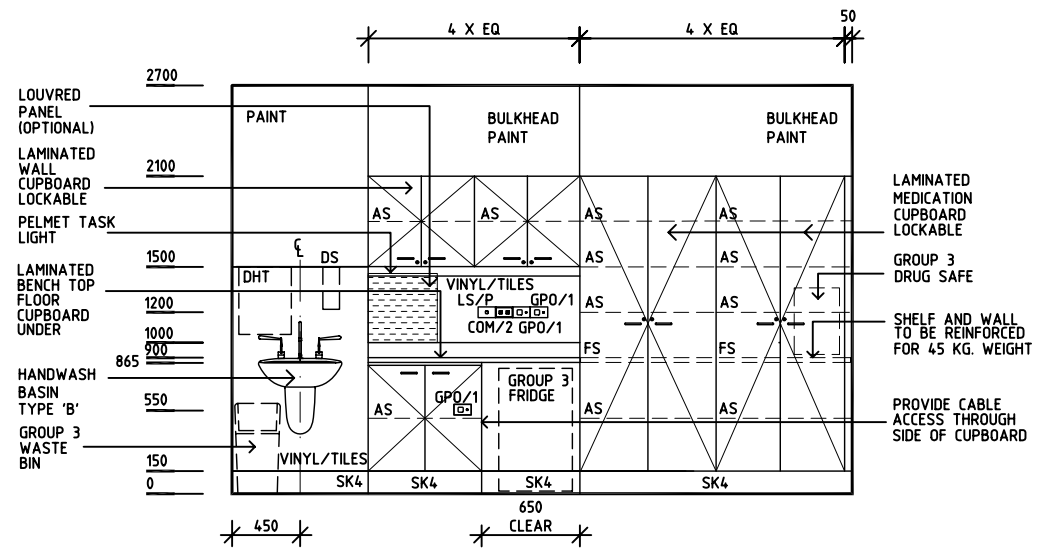
ELEVATION 4
