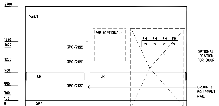
ELEVATION 2
