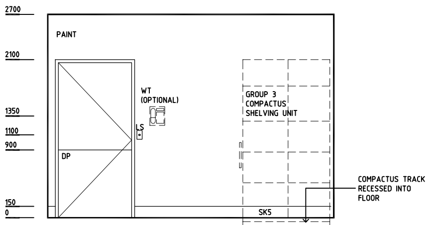
ELEVATION 3
