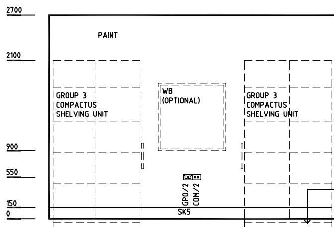
ELEVATION 1
