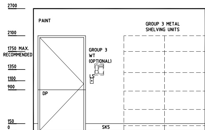
ELEVATION 3
