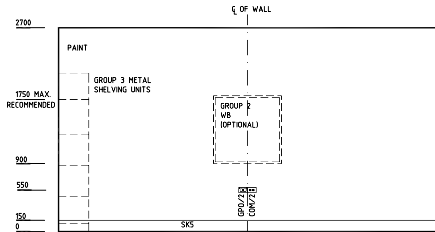
ELEVATION 2
