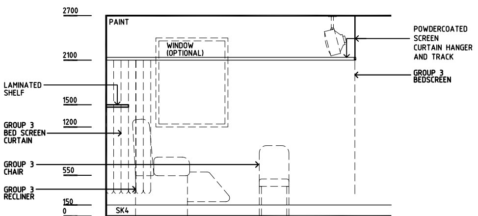
ELEVATION 1
