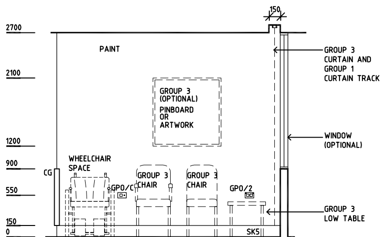
ELEVATION 1
