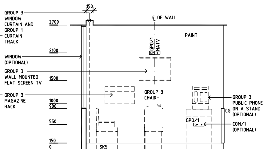
ELEVATION 2
