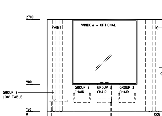
ELEVATION 1
