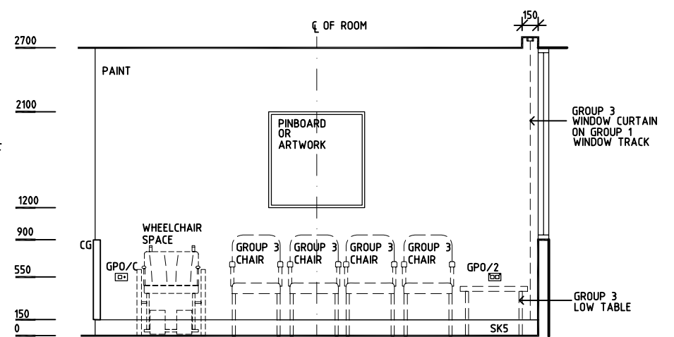
ELEVATION 3
