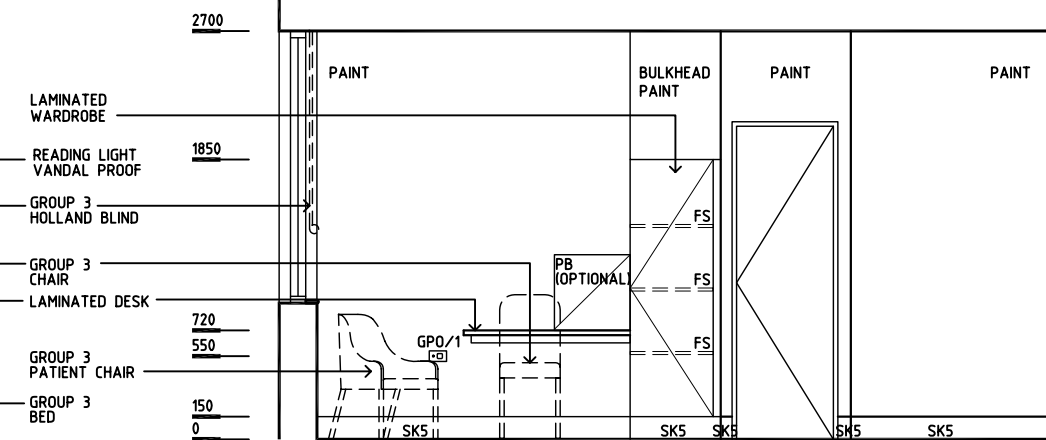
ELEVATION 2
