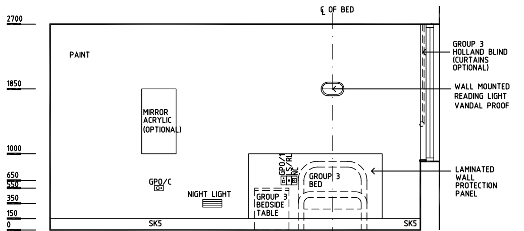
ELEVATION 4
