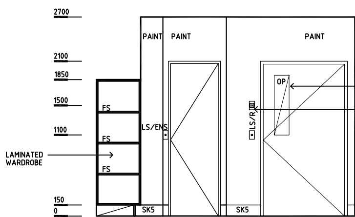
ELEVATION 3
