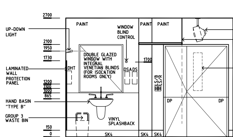
ELEVATION 3
