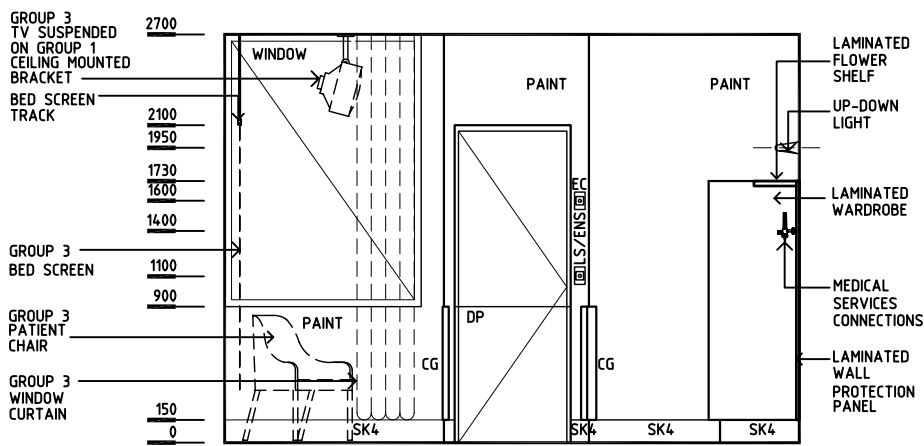
ELEVATION 1
