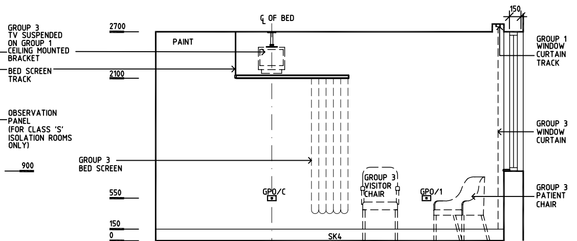
ELEVATION 4
