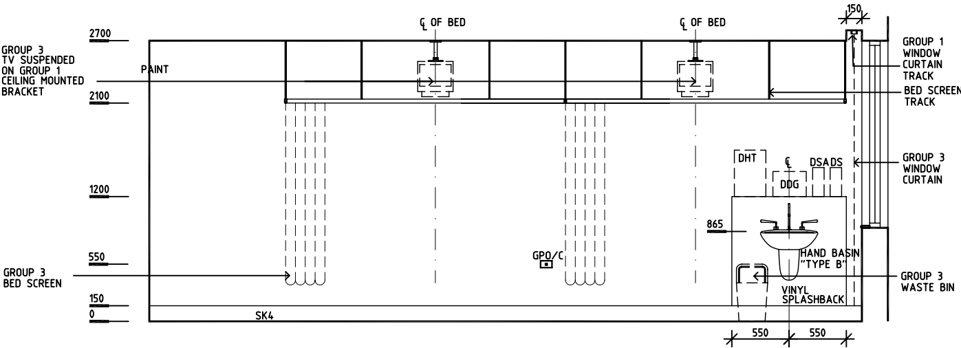
ELEVATION 4
