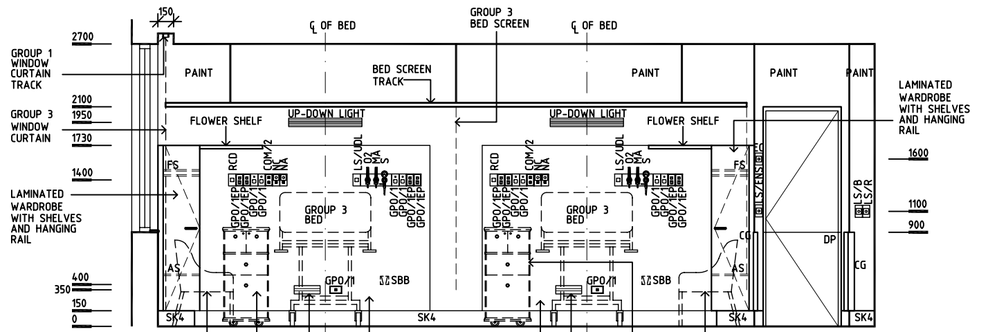
ELEVATION 2
