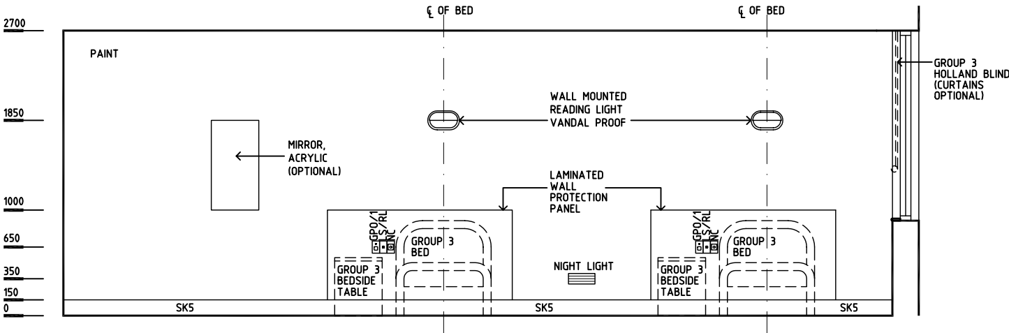
ELEVATION 4
