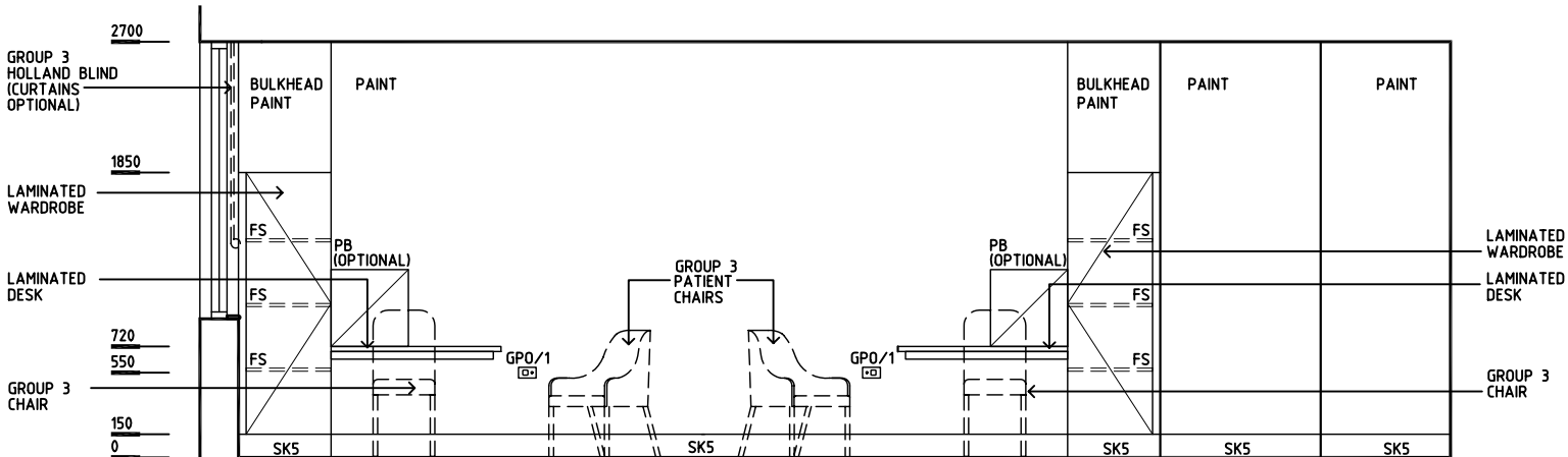
ELEVATION 2
