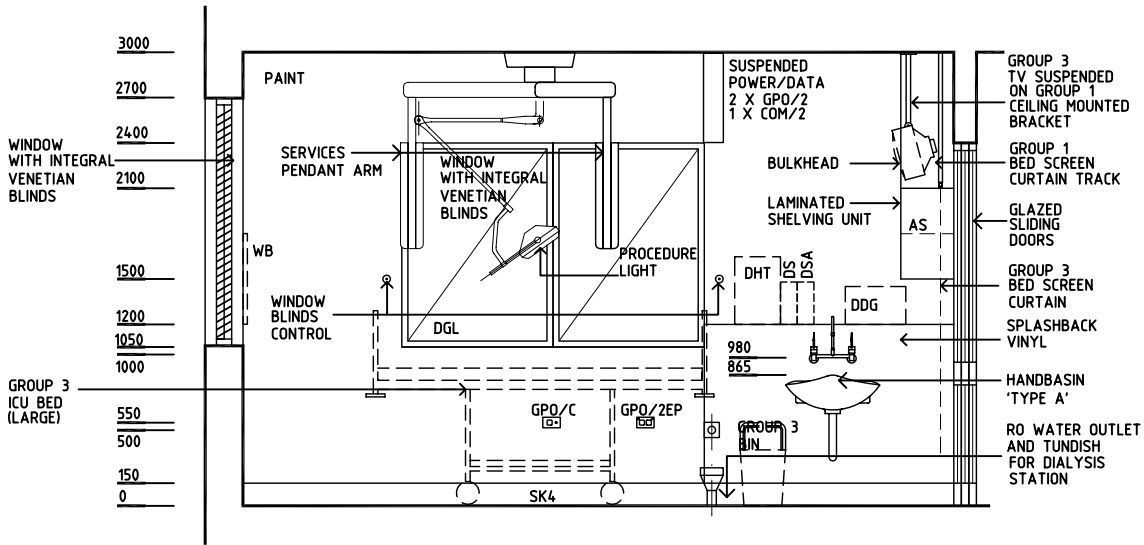
ELEVATION 2
