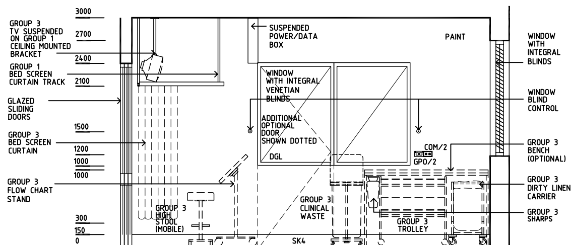
ELEVATION 4
