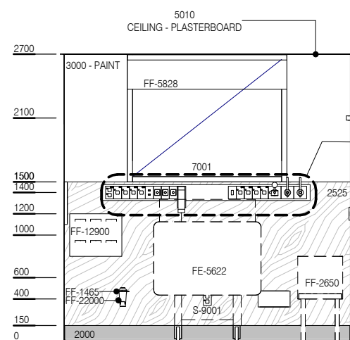
ELEVATION 1
