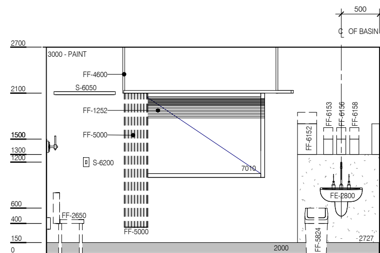
ELEVATION 2
