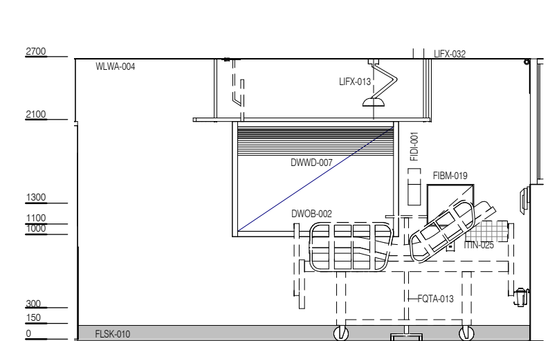
ELEVATION 4
