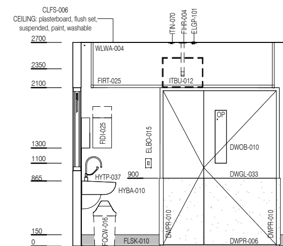
ELEVATION 3
