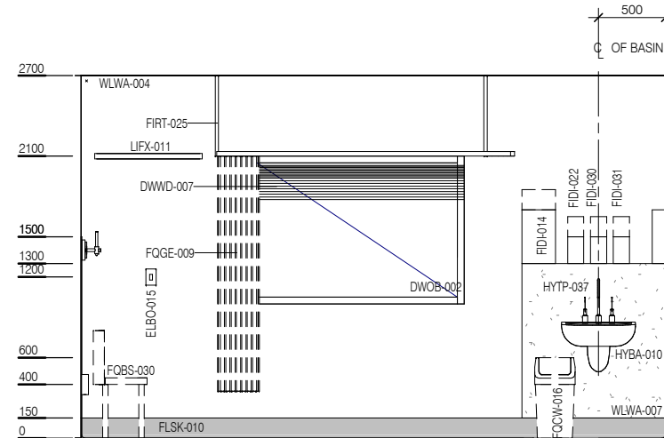
ELEVATION 2
