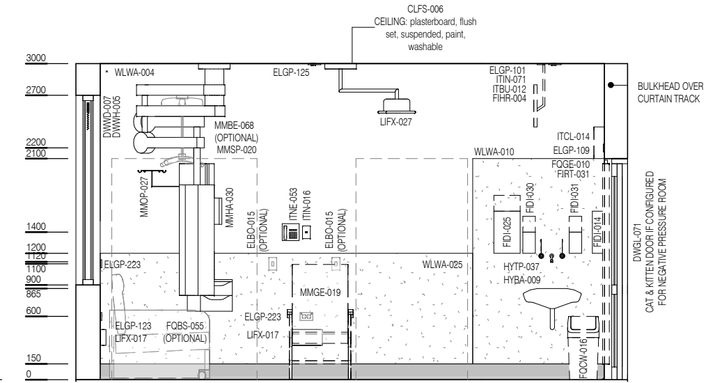
ELEVATION 2
