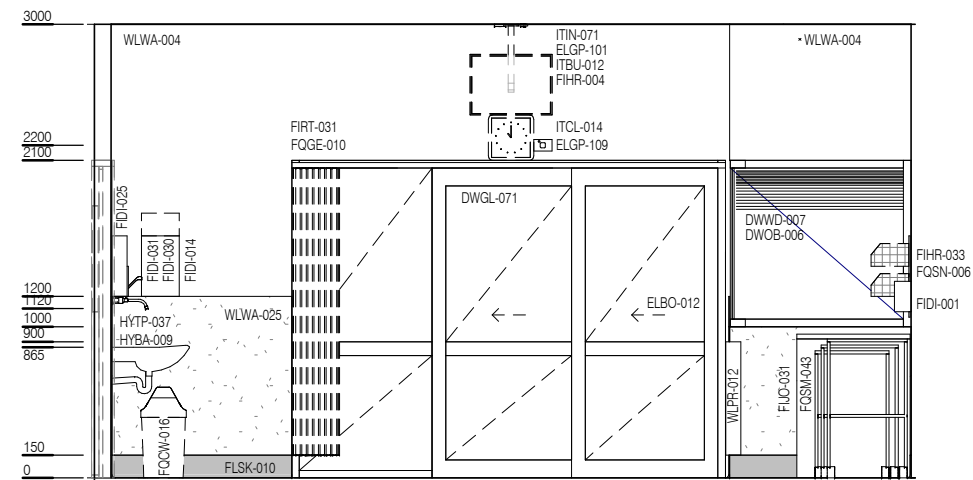
ELEVATION 3
