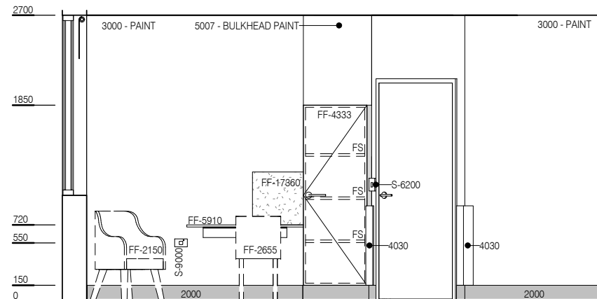
ELEVATION 2
