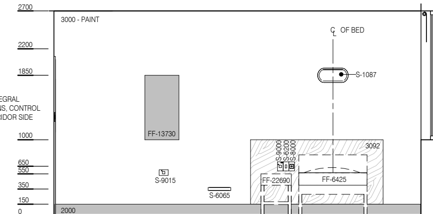
ELEVATION 4
