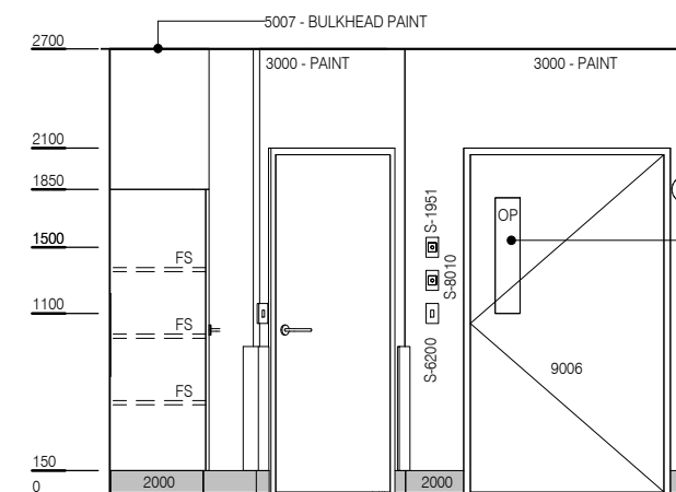
ELEVATION 3
