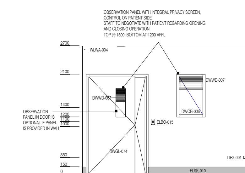
ELEVATION 3
