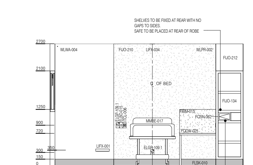
ELEVATION 4
