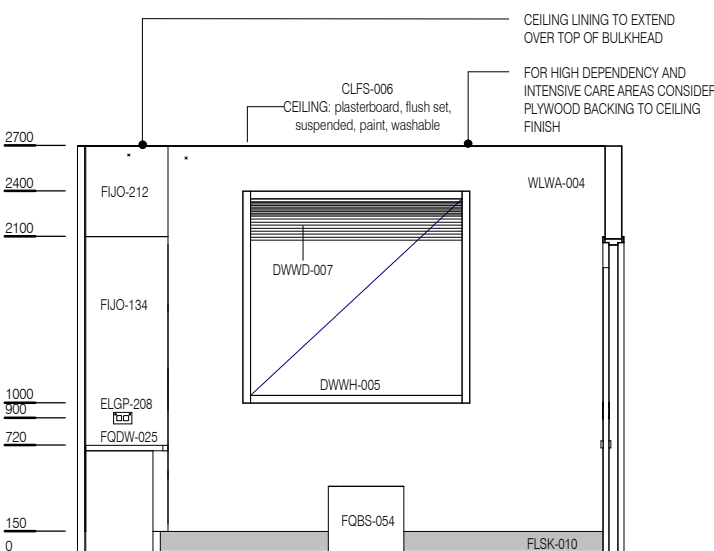
ELEVATION 1
