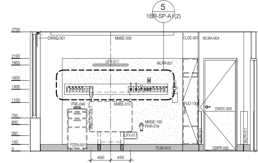
ELEVATION 2
