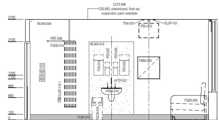
ELEVATION 4
