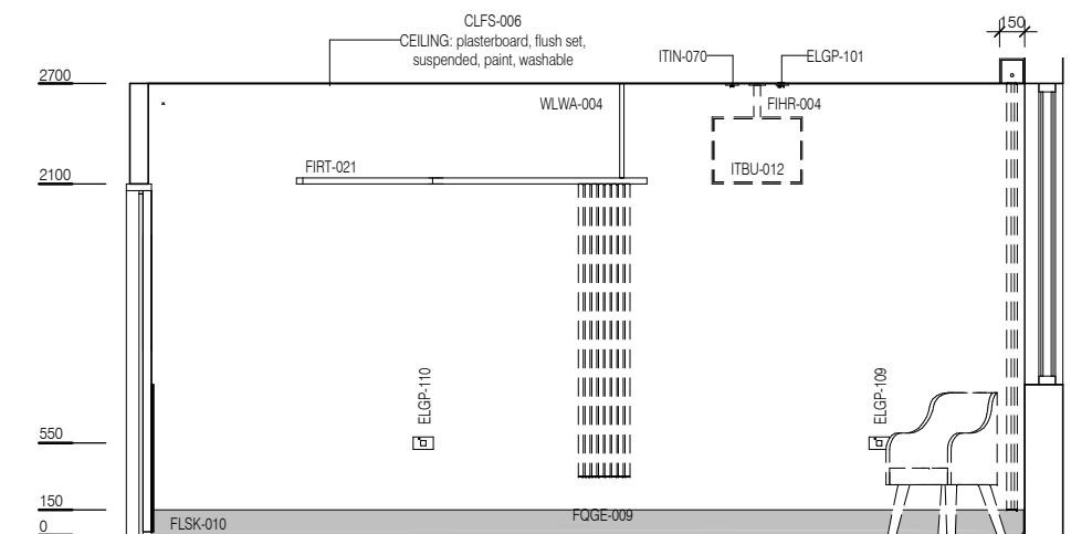
ELEVATION 4
