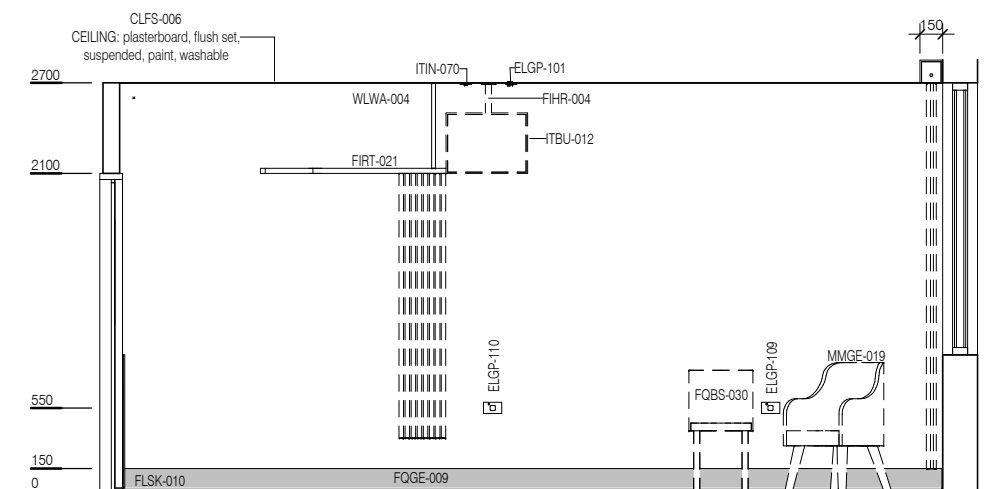
ELEVATION 4
