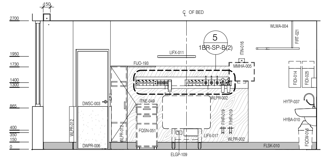
ELEVATION 2
