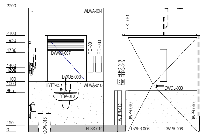
ELEVATION 3
