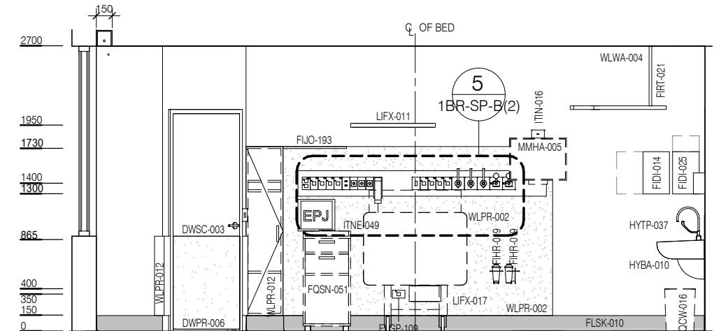
ELEVATION 2
