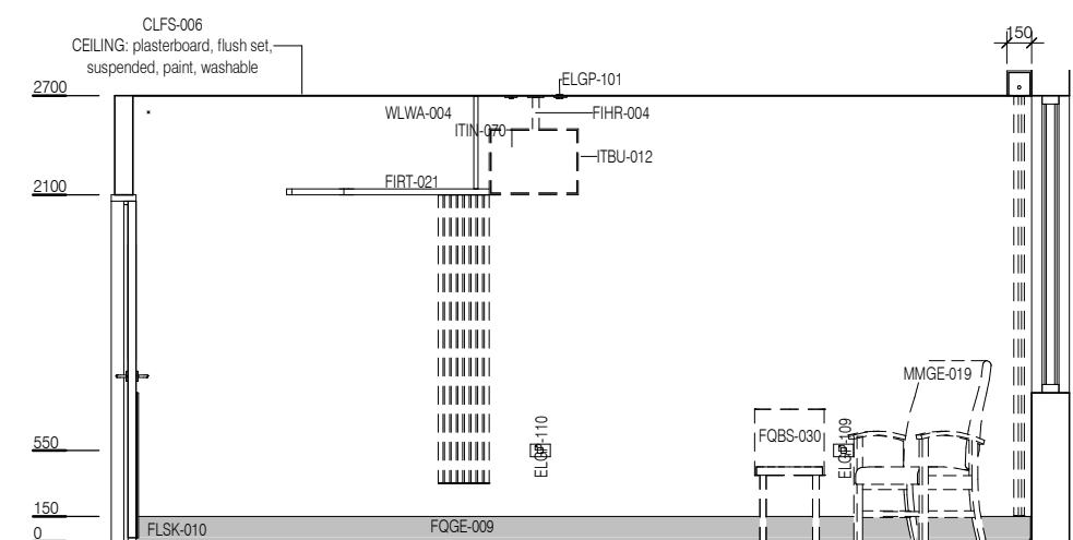
ELEVATION 4
