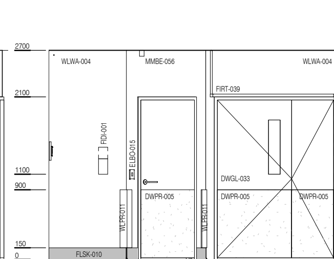
ELEVATION 3
