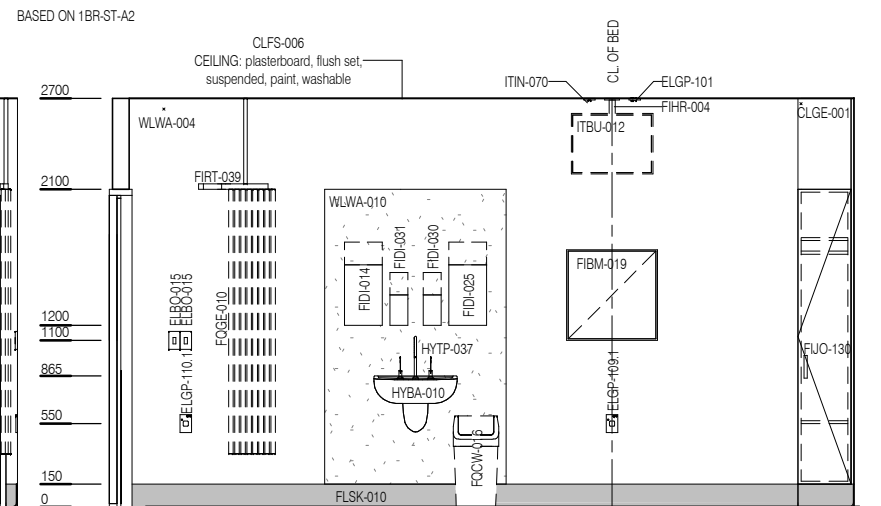
ELEVATION 4
