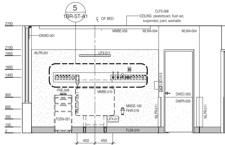
ELEVATION 2
