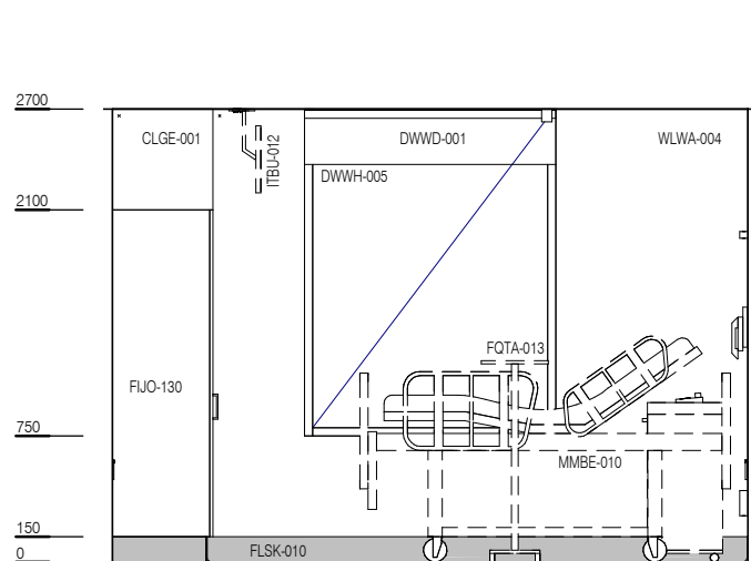
ELEVATION 1
