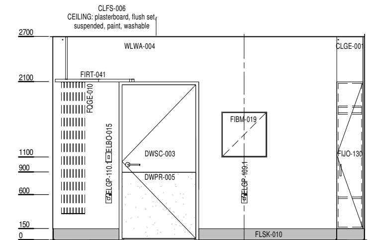
ELEVATION 4
