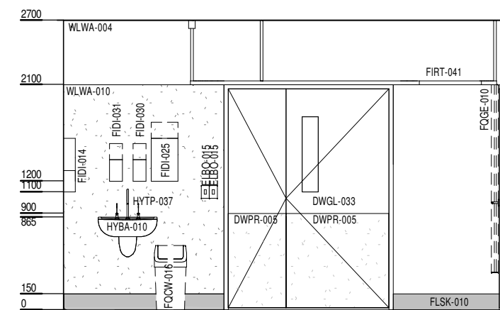
ELEVATION 3
