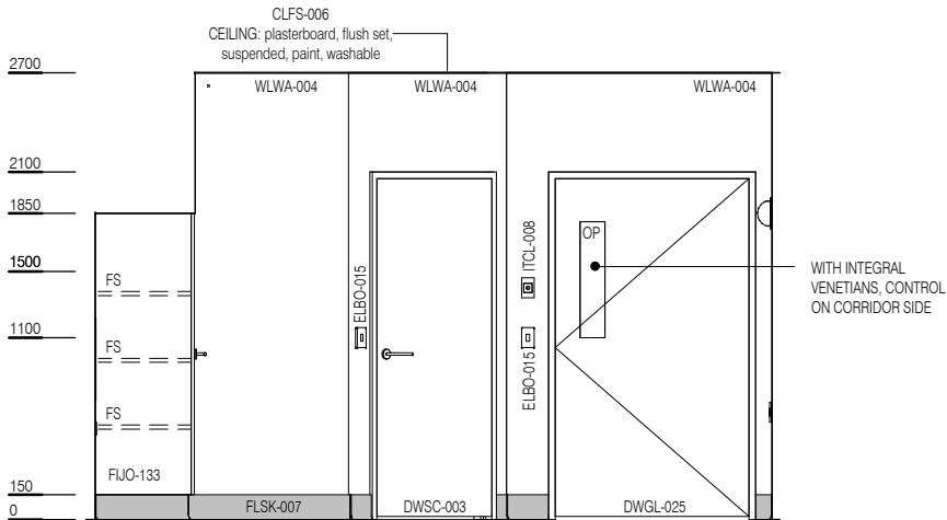
ELEVATION 3
