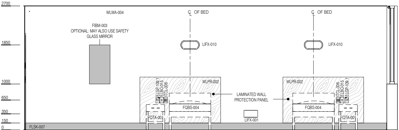
ELEVATION 4
