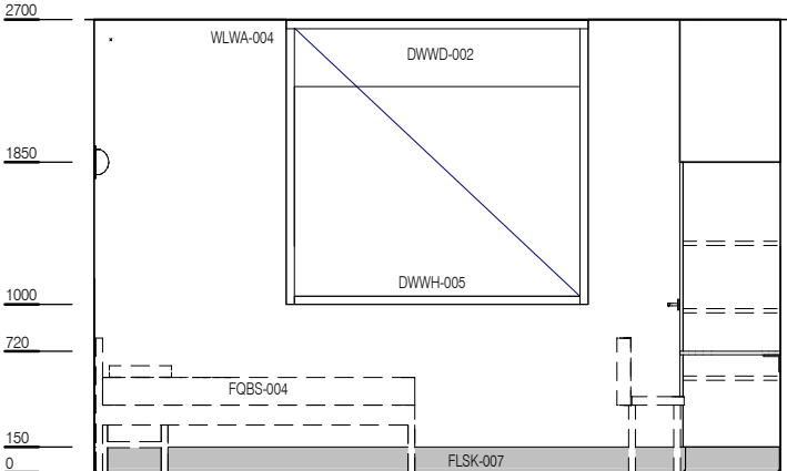
ELEVATION 1
