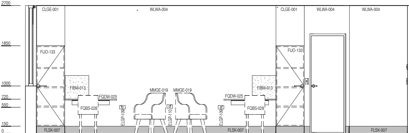
ELEVATION 2
