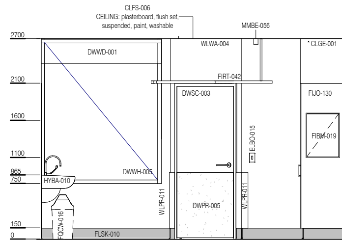
ELEVATION 1
