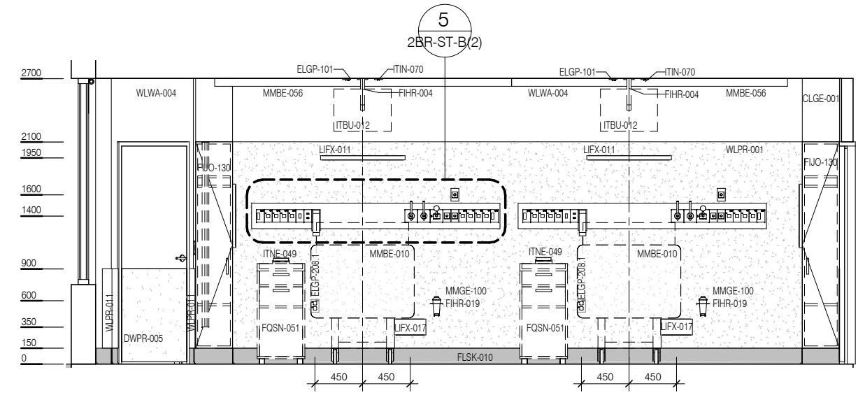
ELEVATION 2
