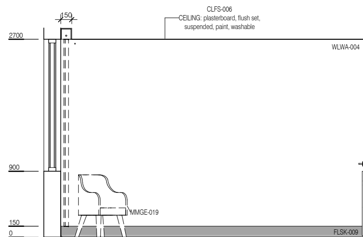
ELEVATION 2
