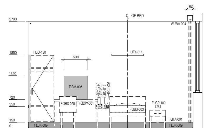
ELEVATION 4
