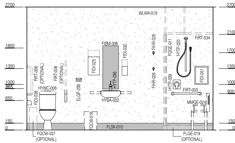
ELEVATION 1
