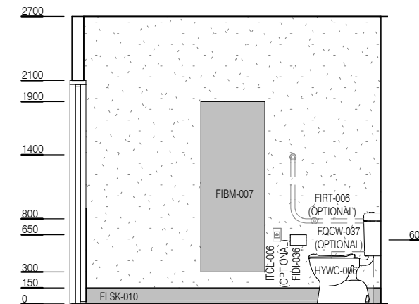
ELEVATION 4
