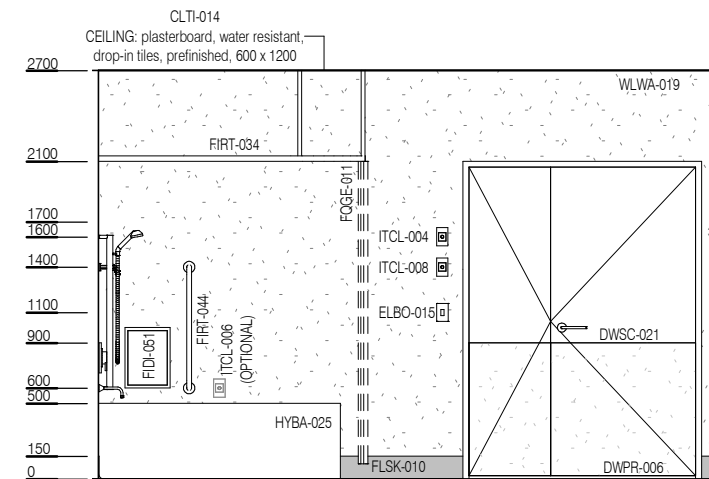
ELEVATION 3
