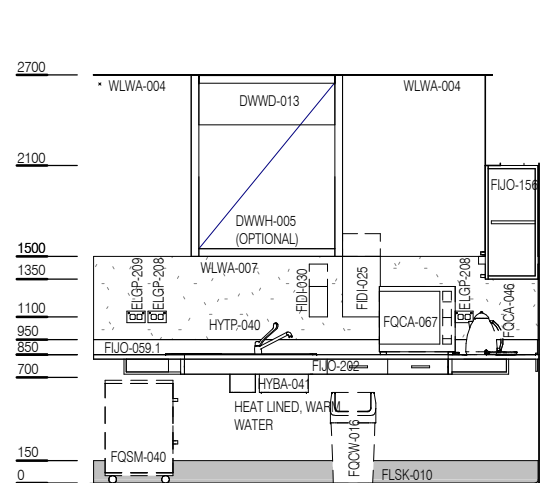
ELEVATION 1
