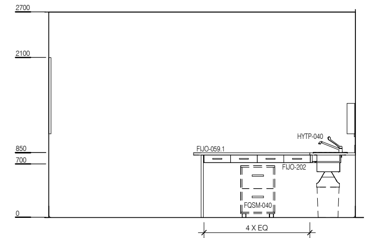
ELEVATION 4
