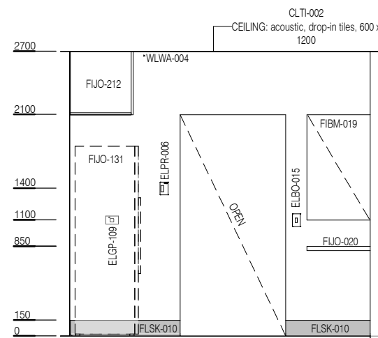
ELEVATION 3
