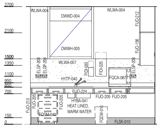
ELEVATION 1
