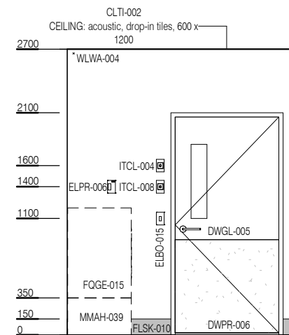
ELEVATION 3
