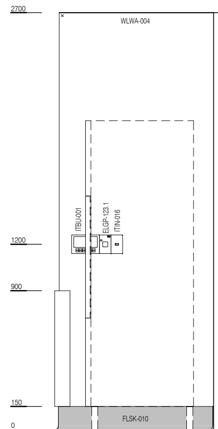
ELEVATION 1
