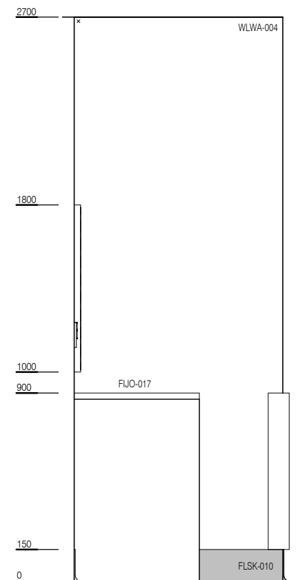
ELEVATION 3
