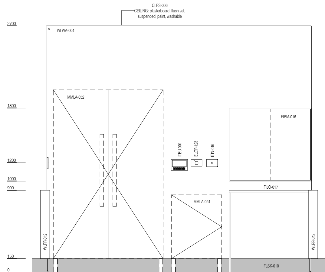
ELEVATION 2
