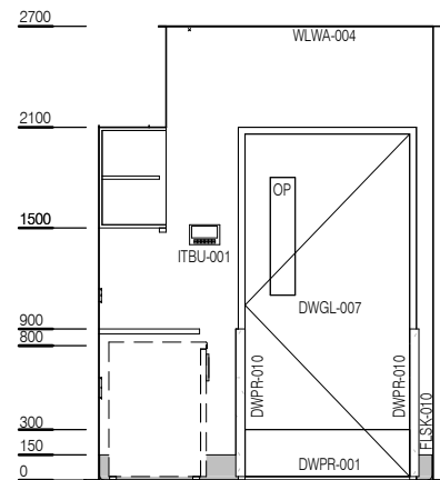
ELEVATION 1
