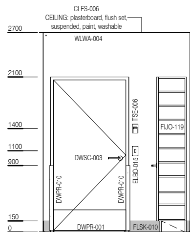
ELEVATION 2
