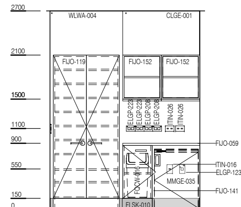
ELEVATION 3
