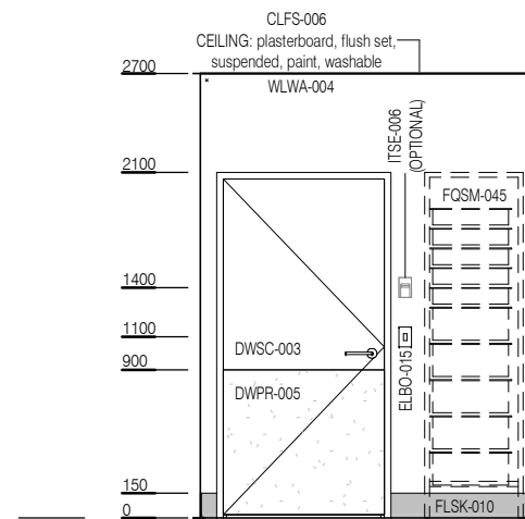
ELEVATION 2
