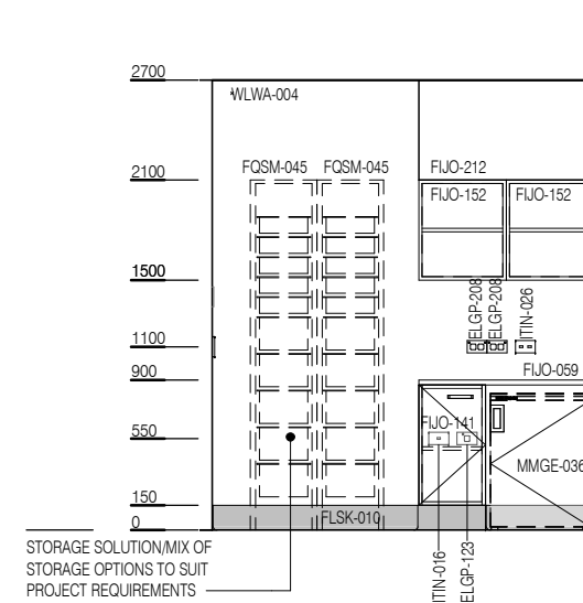
ELEVATION 3
