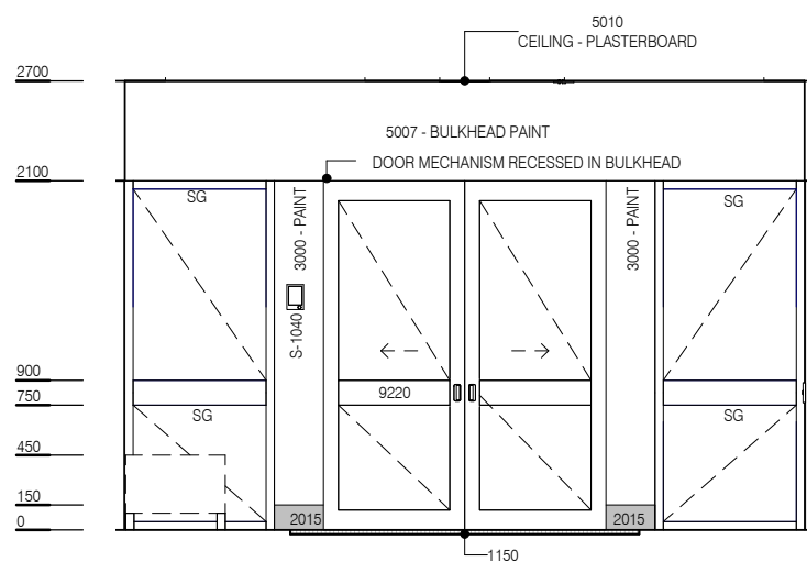
ELEVATION 1
