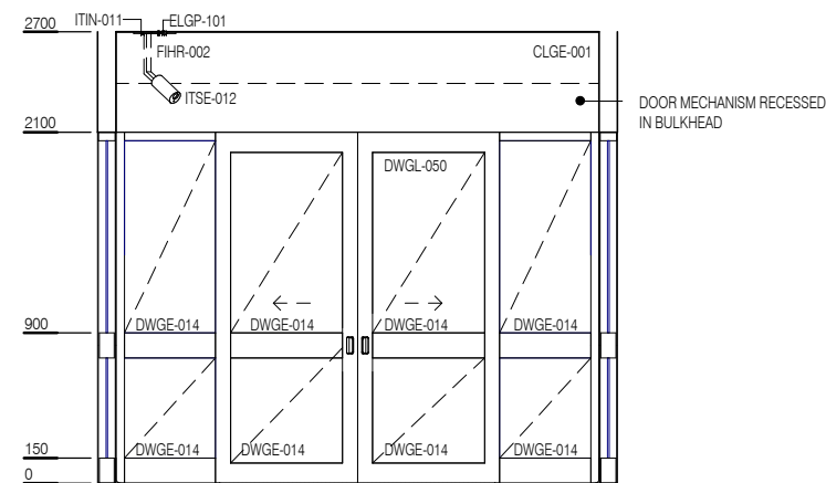
ELEVATION 1
