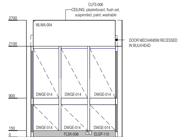
ELEVATION 2
