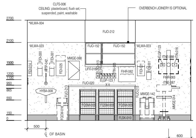
ELEVATION 2
