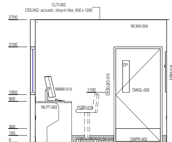
ELEVATION 3
