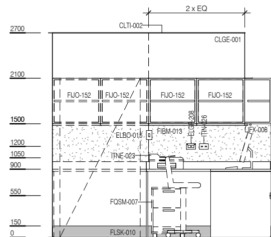
ELEVATION 1
