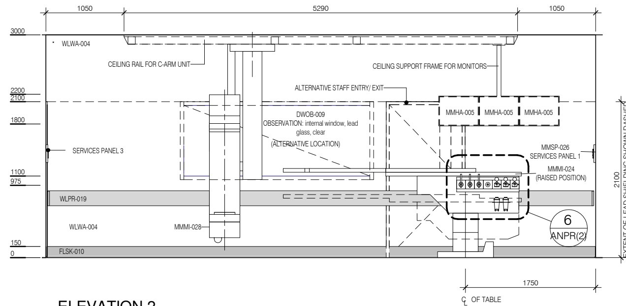
ELEVATION 2
