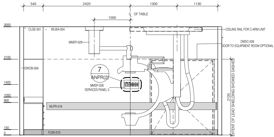
ELEVATION 1
