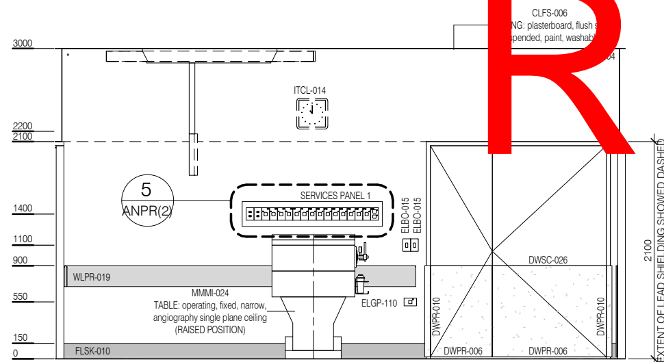
ELEVATION 3
